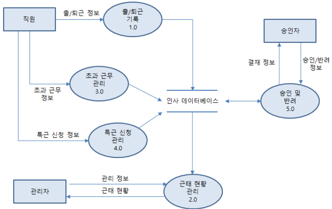
[그림 3-2] 레벨(Level) 0의 자료 흐름도 예시
