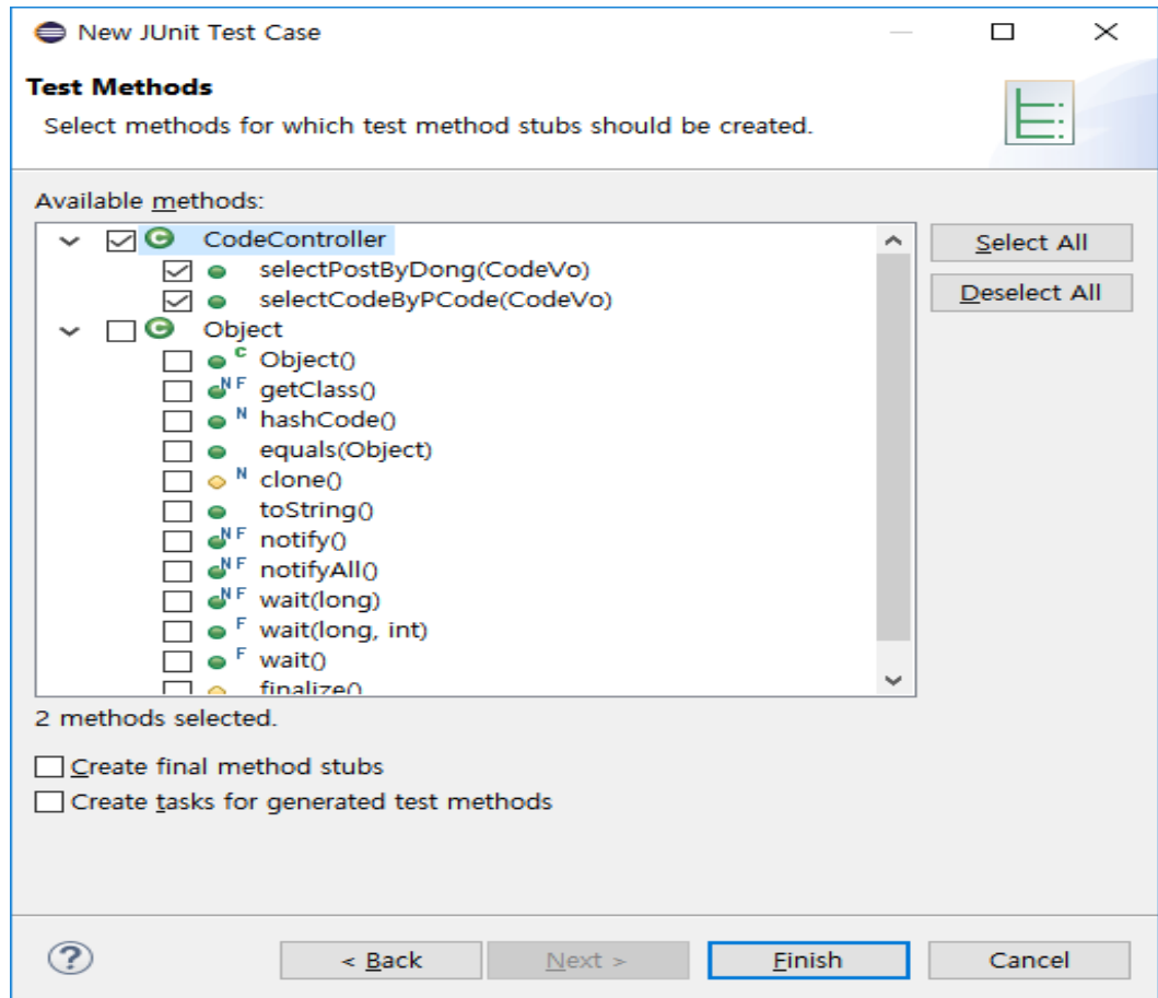
[그림 3-24] 우편번호 조회 단위 테스트 케이스 함수 선택 화면 예시
