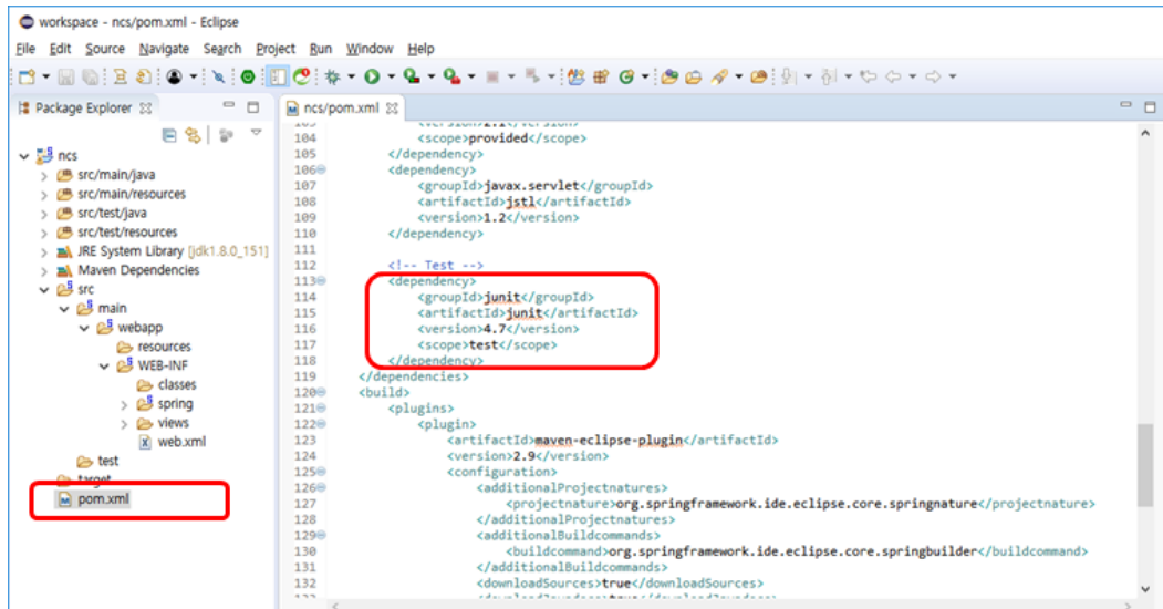
[그림 1-15] 단위 테스트 도구 설치 확인 화면 예시
