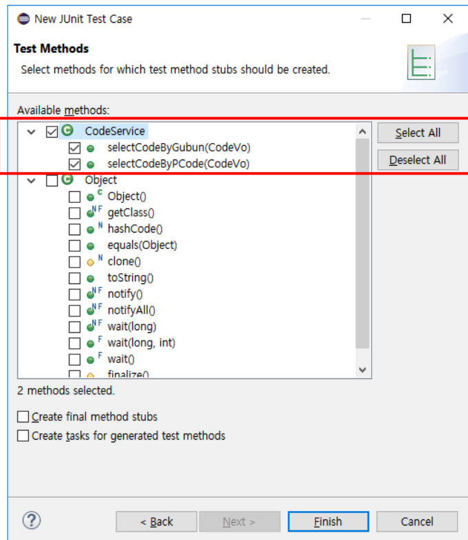
[그림 2-20] 테스트 케이스 생성 시 함수 선택 예시
