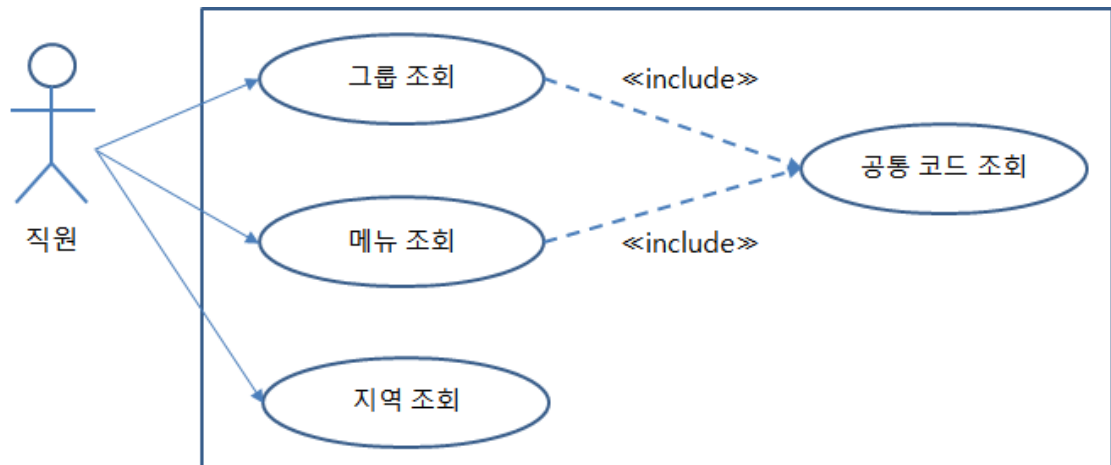
[그림 2-15] 공통 모듈로 식별된 유스 케이스 참고 예시
