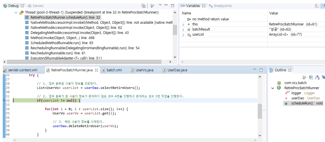
[그림 4-14] 중단점이 지정된 코드에서 실행이 중단된 화면 예시
