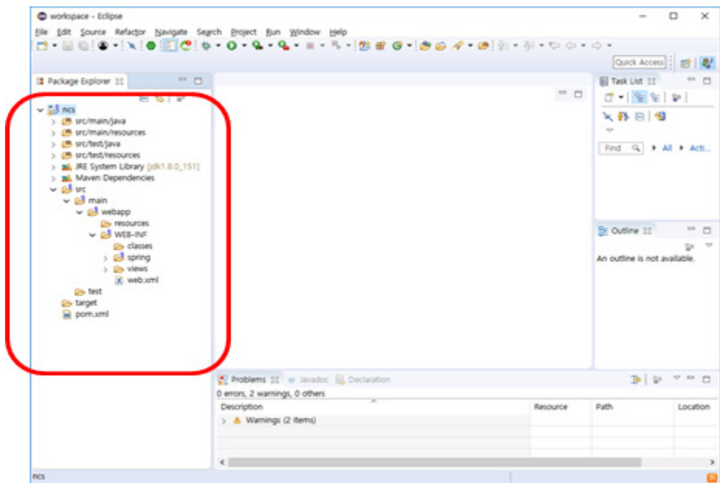
[그림 1-14] Maven 기반의 Spring 웹 프로젝트 구성
