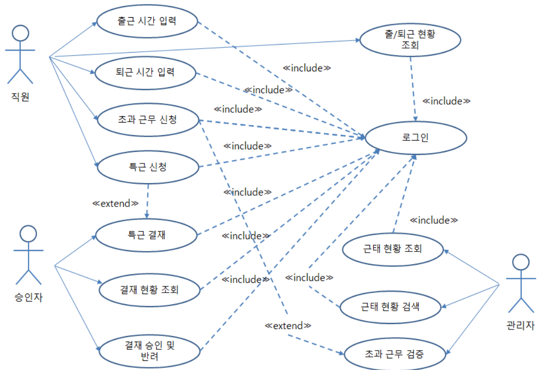
[그림 3-3] 사용 사례 다이어그램 예시
