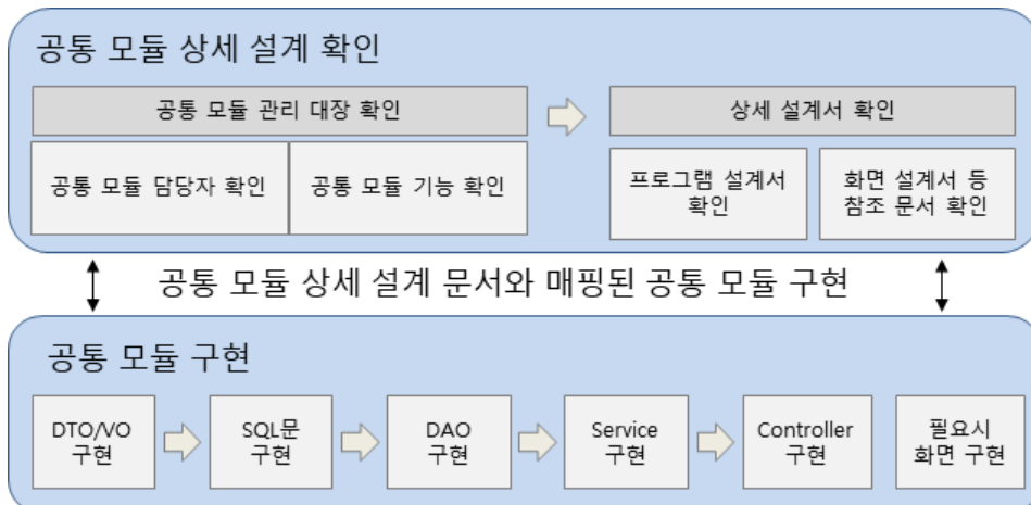
[그림 2-3] 공통 모듈 상세 설계를 기반으로 공통 모듈 구현 순서
